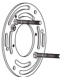
1- Mounting Plate (D)
