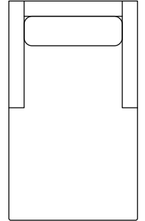
CHAISE 35"H x 36¼"W x 57"L •US279
